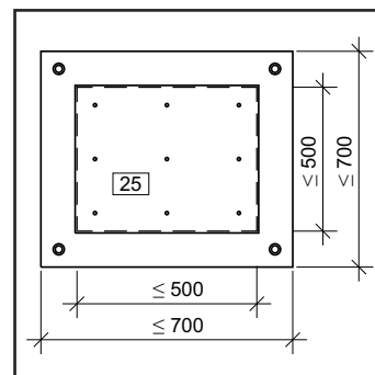
[22] Zugangsklappe
