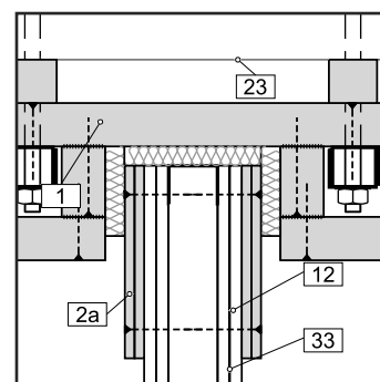
[19] Wandschneidung Variante
