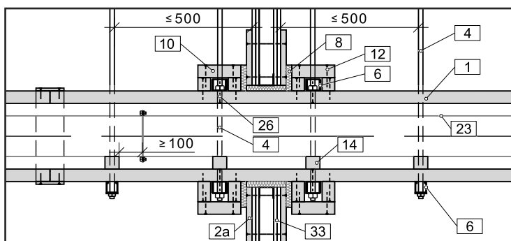
[18] Wandschneidung durch Leichtbauwand
