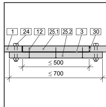
[24] Schnitt Zugangsklappe
